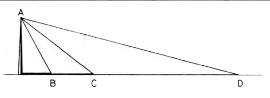
Şema 1: BAC açısı CAD açısıyla eşittir; fakat BC doğrusu CD doğrusu ile eşit değildir.
